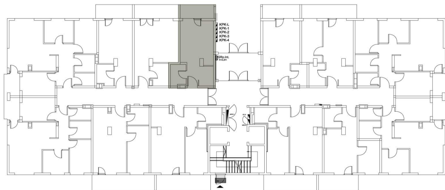
Osnova sprata
